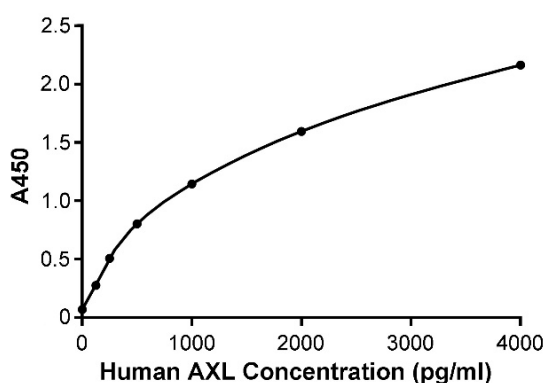
图3. Human AXL ELISA Kit的标准曲线。实测数据会因实验条件、检测仪器等的不同而存在差异，图中数据仅供参考。
